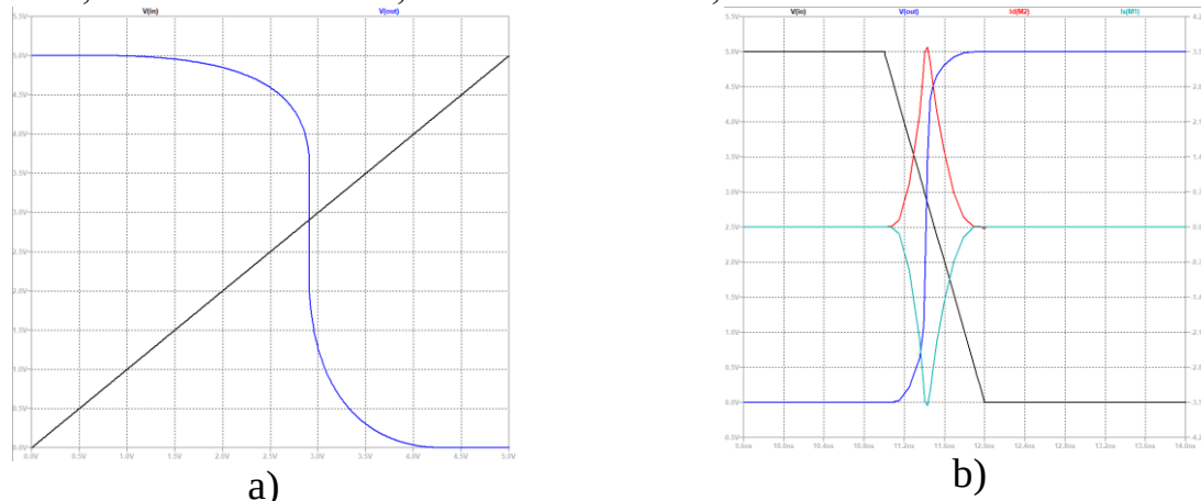
Рис. 2. Моделювання передавальної характеристики (а) та моделювання перехідних процесів (б)
